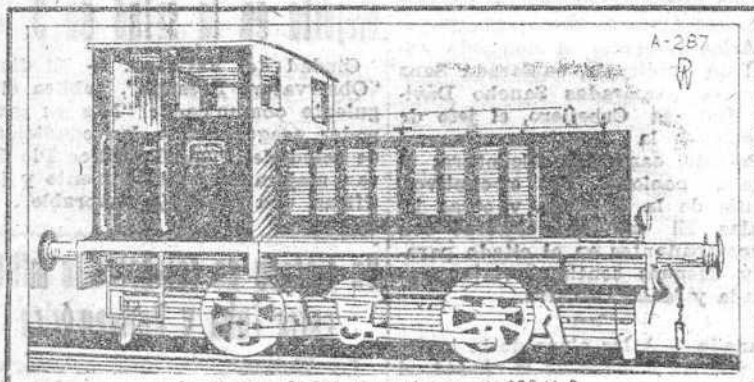
Locomotoras Diesel de manobras, de 100 H.P.
