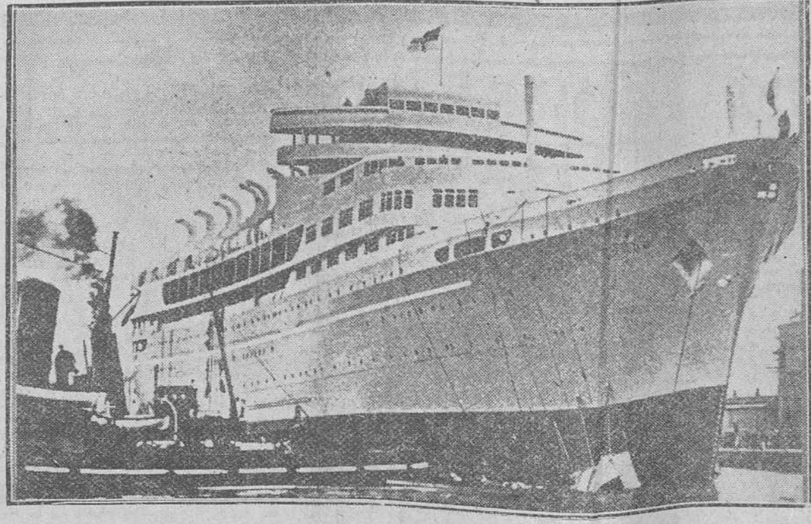
Una vista del nuevo navío británico de 22.000 toneladas "Cruz del Sur", después de su botadura por la Reina Isabel en Belfast. "El Cruz del Sur" es el primer gran barco de pasajeros que lleva las máquinas a popa, en vez de en medio del buque; tiene cabida para 1.200 pasajeros a todo confort y puede hacer cuatro viajes alrededor del Mundo, cada año. La Reina lo calificó de "algo enteramente nuevo y original".—(F. Gil del Espinar)
