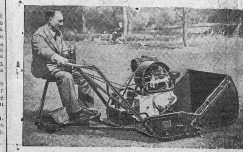
En una reciente demostración de la Real Sociedad Británica de Horticultura se exhibió este modelo de máquina segadora "Dennis" accionada por un pequeño motor que lleva debajo del asiento un rodillo adicional. (Foto Calpe)
