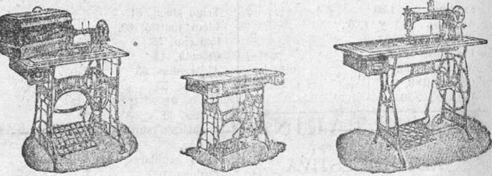
Máquina doméstica, cose hacia adelante y hacia atrás. 250 pesetas. Máquina secrete, de lanzadera vibrante. 325 pesetas. De bobina central 395 pts. Máquina industrial, fuerte y silenciosa a 400 pesetas. Bobina central
