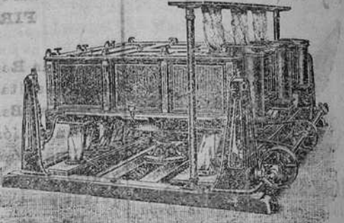
PLANSICHTER (último modelo) -- Construcción Daverio.
