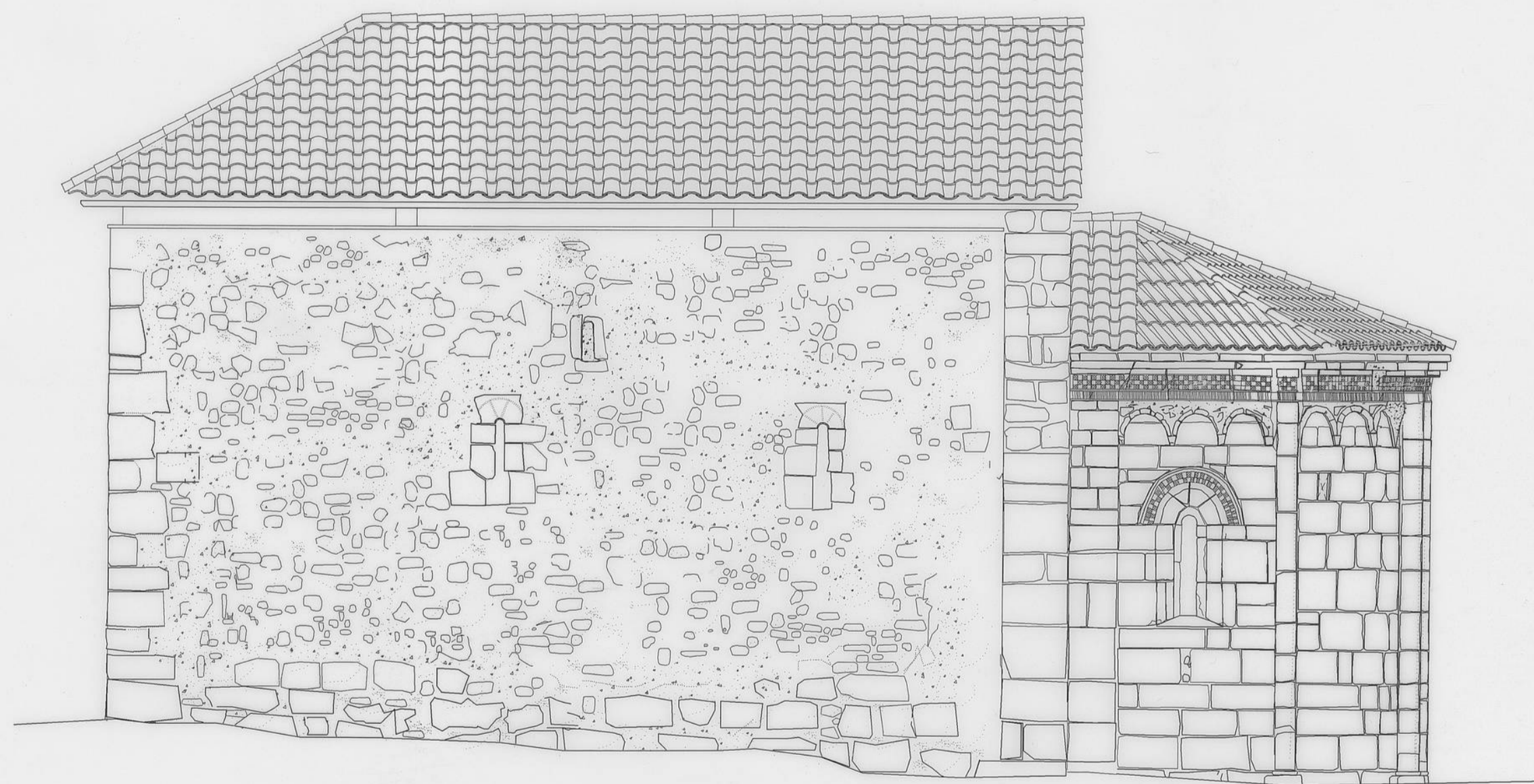
ALZADO SUR
