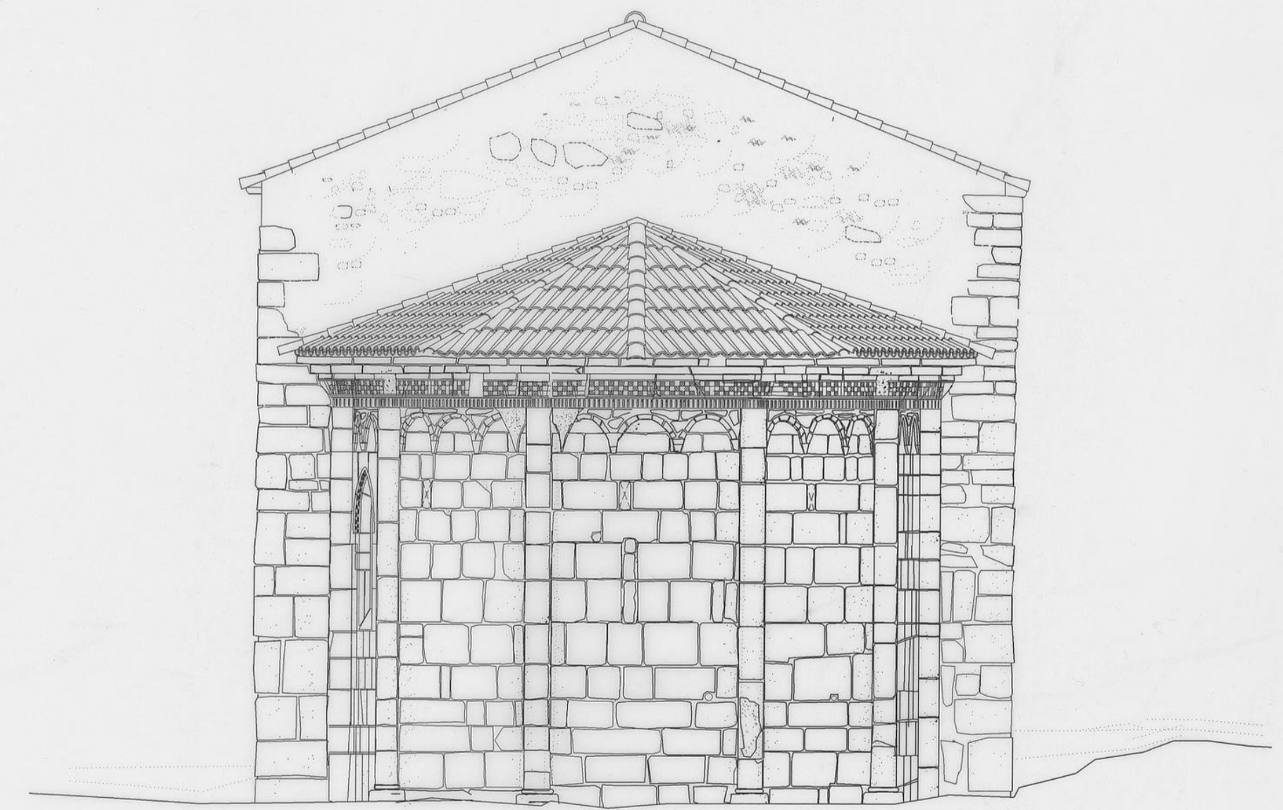
ALZADO ESTE
