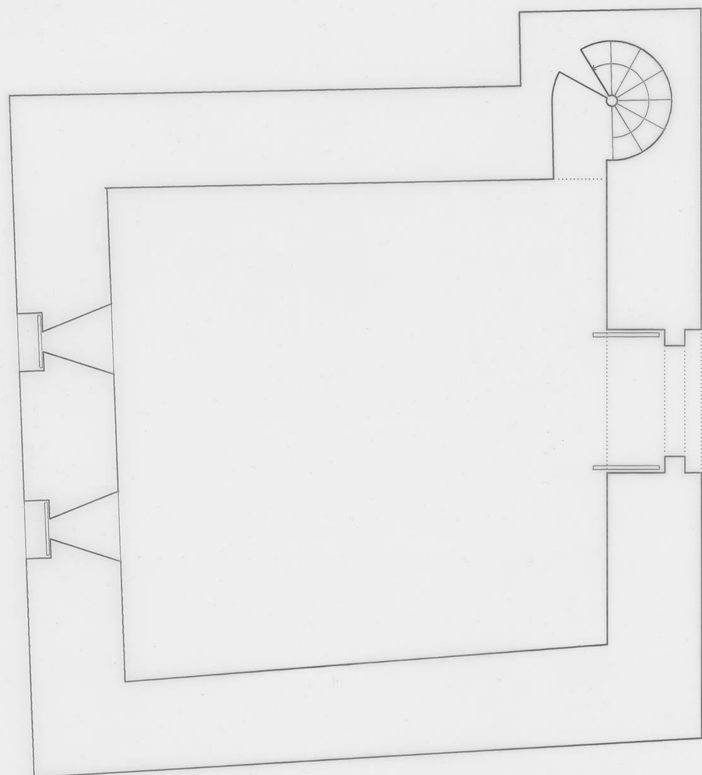
PLANTA BAJA
