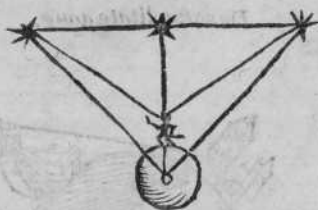
Stella super caput nostrum.
