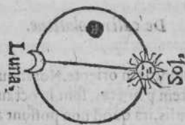
Figura qua declarat non posse fieri eclips. Lunæ, si terra non est in medio mundi.
