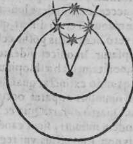
Directus.
