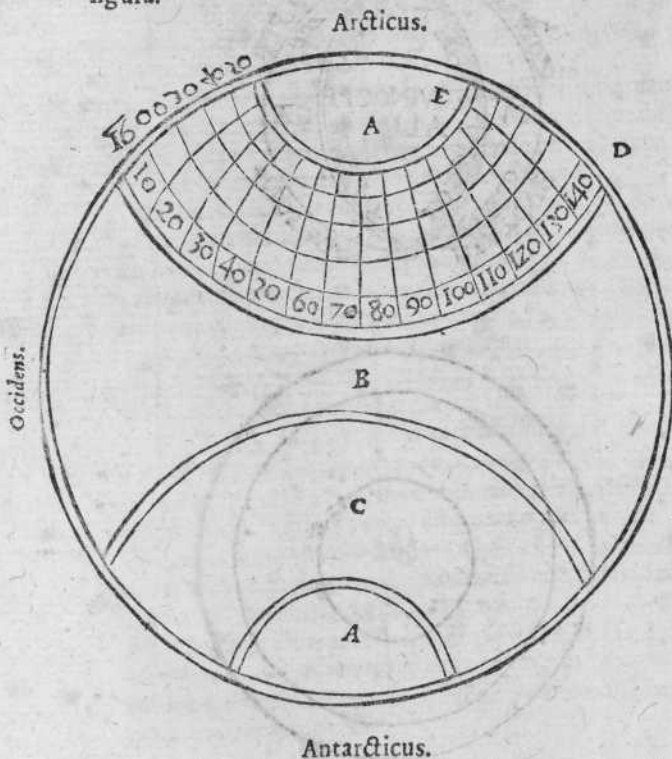
A Mare. B Circulus descriptus in superficie terræ correspondens æquinoctiali. C Terra australis, incognita secundum Ptolomæum. D Lineæ latitudinum ab oriente ad occidentem ductæ. E Lineæ longitudinum ab arctico ad æquinoctialium ductæ.
