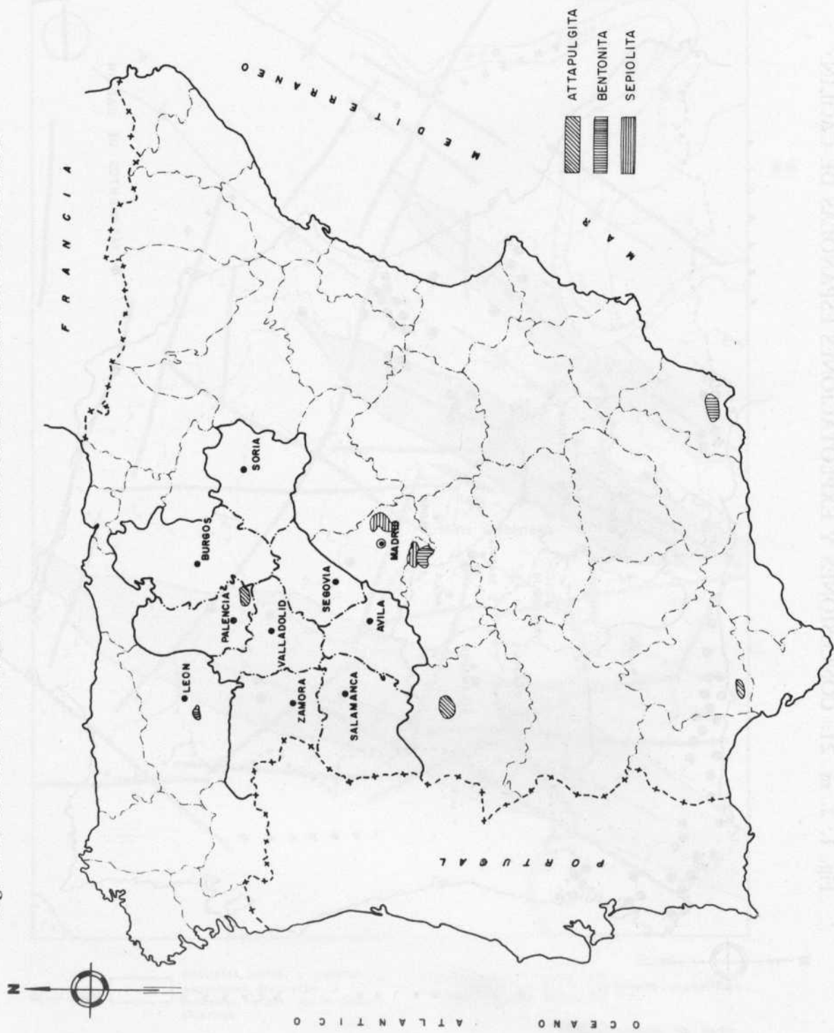
Fig. 1. 2. m. 22: YACIMIENTOS ESPAÑOLES DE ARCILLAS ESPECIALES
