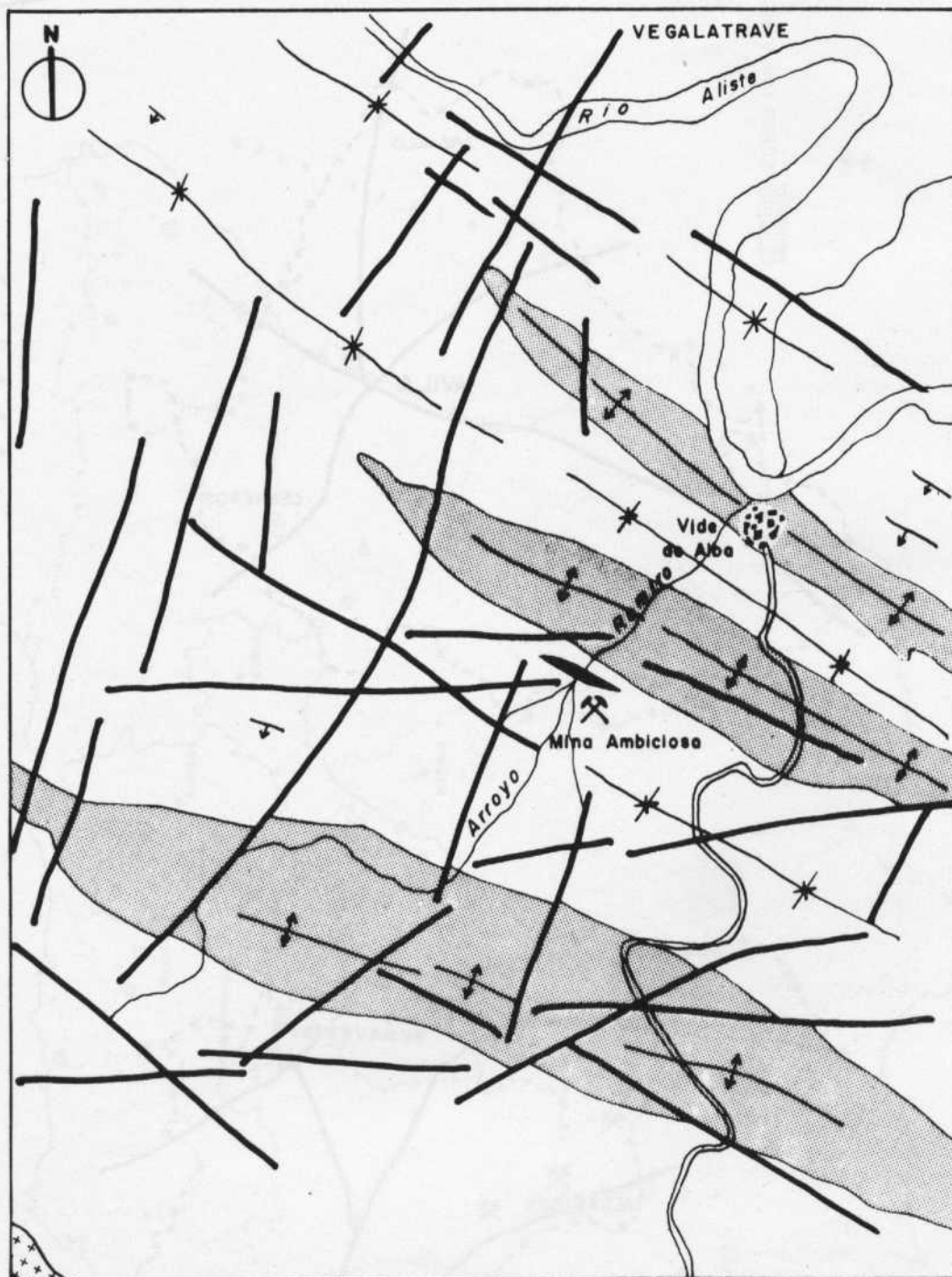
Fig. I. 2. m. 20: SITUACION GEOLOGICA DE LA MINA «AMBICIOSA» EN VIDE DE ALBA (ZAMORA)
