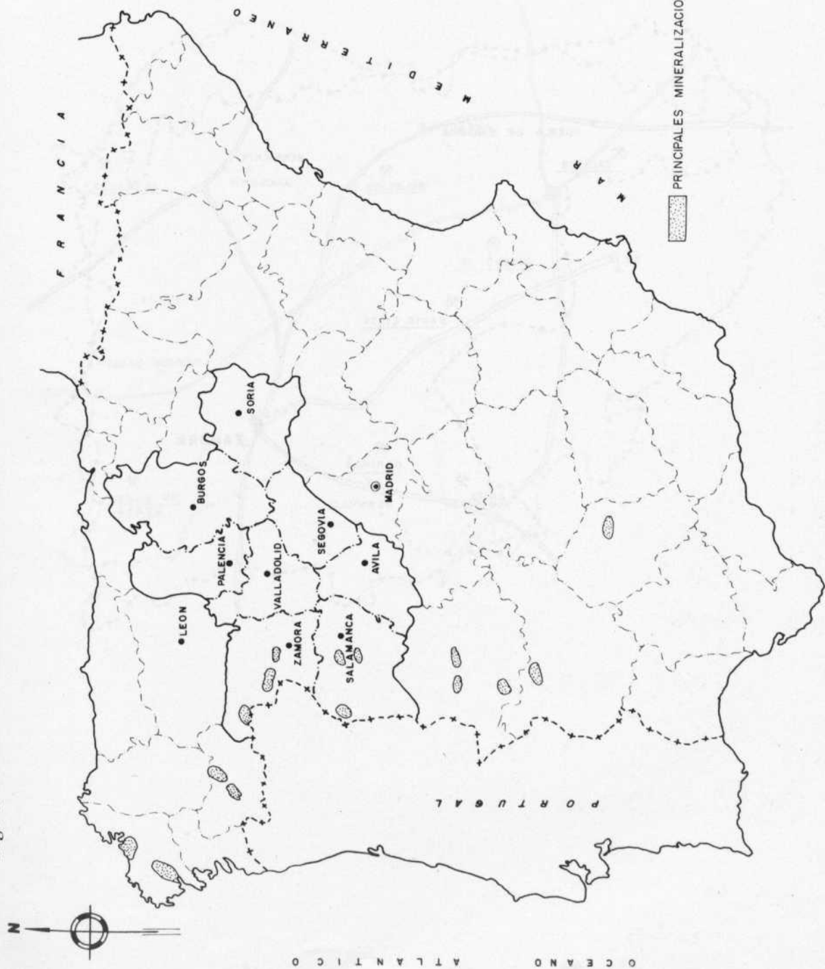
Fig. I. 2. m. 15: PRINCIPALES ZONAS ESPAÑOLAS CON MINERALIZACIONES DE ESTAÑO
