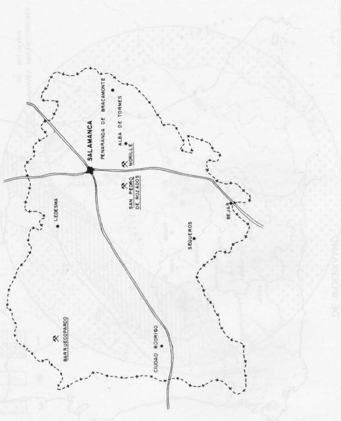
Fig. I. 2. m. 12: PRINCIPALES YACIMIENTOS DE WOLFRAMIO DE LA PROVINCIA DE SALAMANCA
