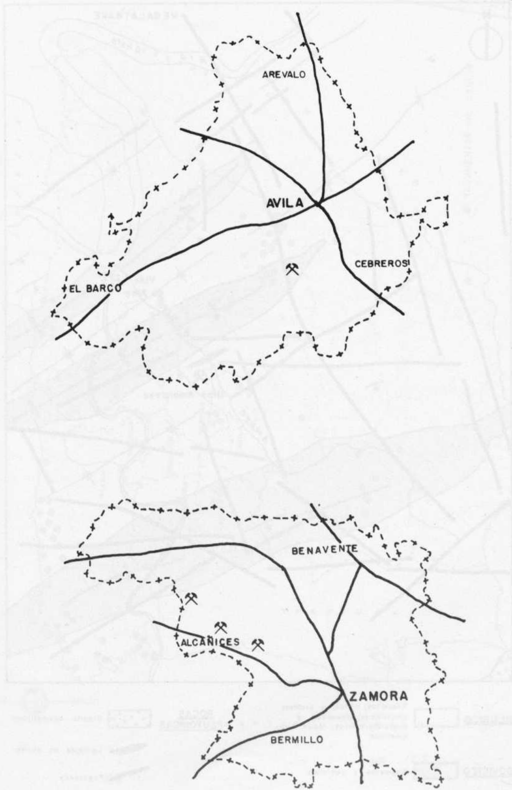
Fig. I. 2. m. 19: SITUACION DE LOS YACIMIENTOS DE BARITA EN LAS PROVINCIAS DE AVILA Y ZAMORA
