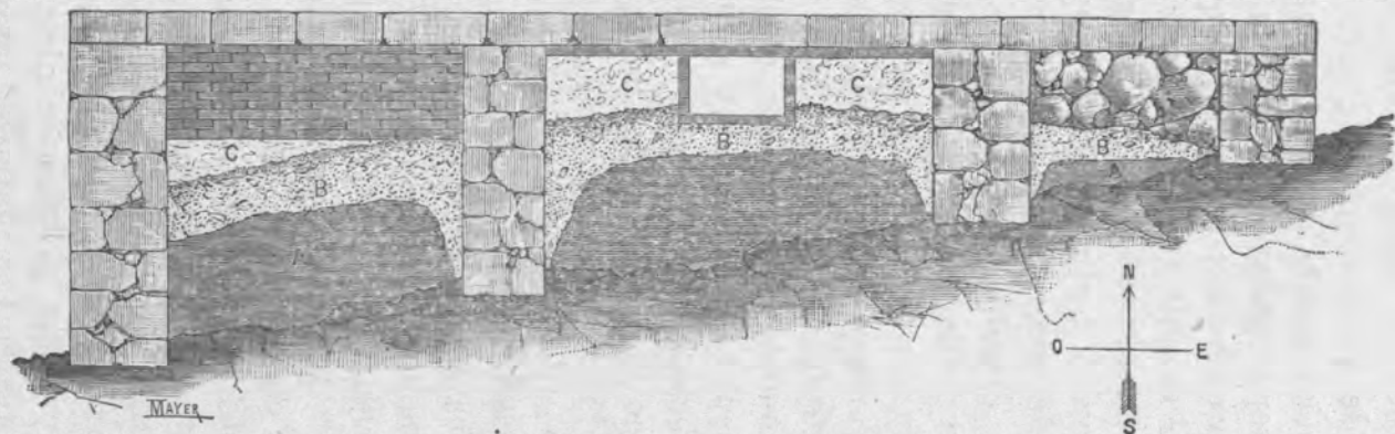
Corte longitudinal del basamento del mausoleo de Santiago. Las letras A, B, C, indican las tres capas sobrepuestas que rellenaban y macizaban los espacios que quedaban entre los muros de los cimientos.
