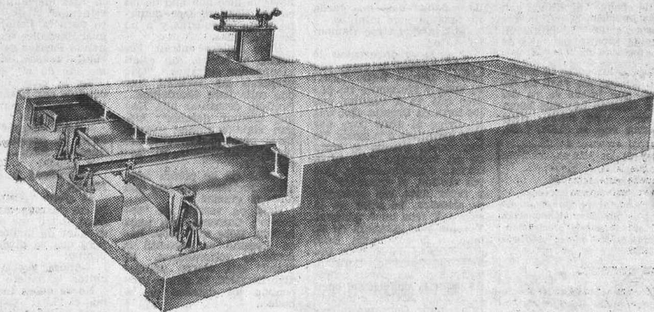
(BASCULA PUENTE PARA PESAR CAMIONES TIPO CM 3.800)
