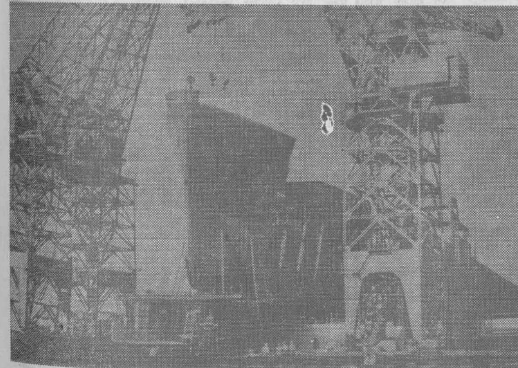
Montaje de una proa prefabricada en grada, en los astilleros de Cádiz. — (Foto LOGOS)
