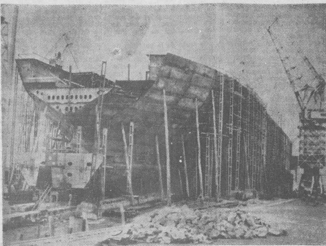
En los astilleros Astano de La Coruña se está construyendo el mayor petrolero de España, el «Ceuta», de 91.000 toneladas. Dicho buque irá equipado con un sistema complejo de mando auto-eléctrico, dotado con su brújula giroscópica. En la foto, vista del futuro petrolero en plena construcción (Foto CIFRA)
