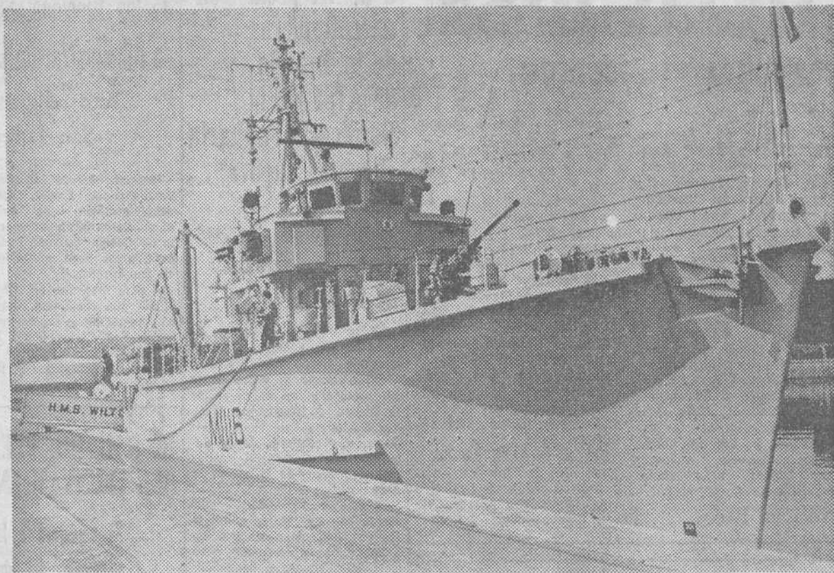
Gran Bretaña cuenta ya con su primer buque de guerra, el «H.M.S. Wilton», un caza-minas con casco de fibra de vidrio reforzado con plástico. El mantenimiento del buque es mínimo debido a su resistencia a la corrosión. El buque fue construido en 1972 y, después de un largo período de pruebas, ha recibido el visto bueno de los expertos. — (Foto FIEL).
