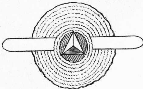
Núm. 5. Puya y tope del nuevo modelo visto de frente.
