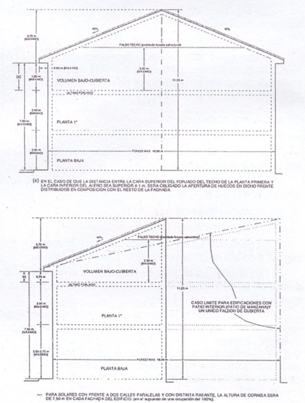
GRAFICO N.º 1 ZONA A. REGULACION DE LA ALTURA DE LA EDIFICACION
