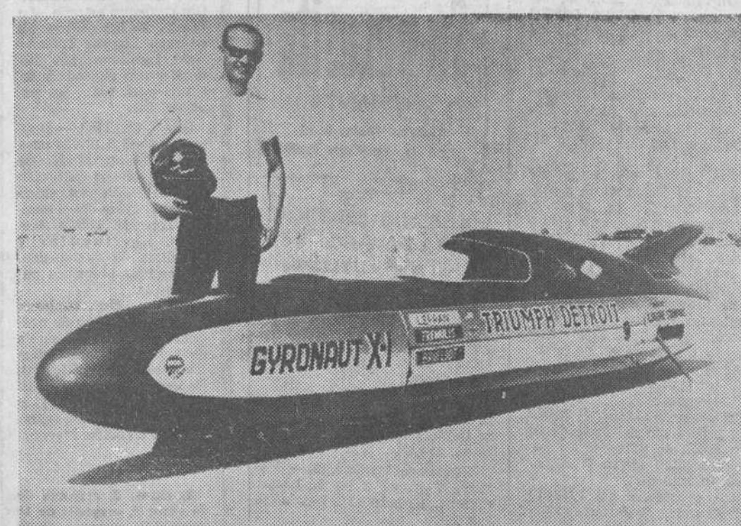
Bob Leppan, de Detroit, Estados Unidos, aparece en esta fotografía con el «Gyronaut X-1», con el que ha logrado un nuevo record de la Asociación Americana de Motociclistas, al alcanzar una velocidad de 245,667 millas por hora (casi 400 kilómetros), en Donnevill Salt Flats, Estado de Utah. En efecto, el «Gyronaut X-1» es una motocicleta, la más rápida del Mundo, propulsada por dos motores británicos «Triumph» de 650 cc. — (Foto FIEL)
