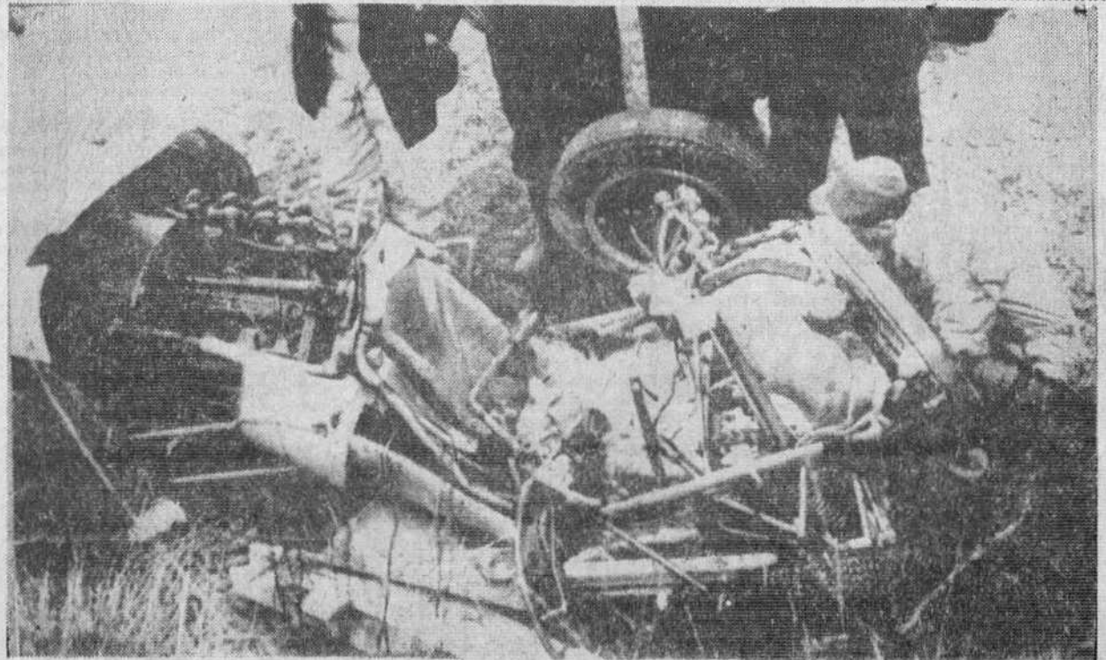
El «Lotus» de Stirling Moss Goodwood (Inglaterra). — Así quedó el bólido «Lotus» que pilotaba el famoso corredor automovilista Stirling Moss, después del accidente sufrido en la carrera que terminó en un informe dicen que el estado de Moss ofrece seria gravedad. El choque contra la barrera protectora se produjo cuando rodaba a 150 kms. hora. — (Foto Cifra)
