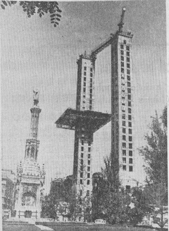
Continúa la construcción de las gigantes torres en la madrileña plaza de Colón. Como se sabe, se trata de dos altos bloques, de los que se ha levantado su estructura central, siguiendo ahora la construcción del resto de los edificios, según el sistema denominado «método del paraguas», empleado por vez primera en España. La foto muestra el estado actual de las obras. — (Foto FIEL).
