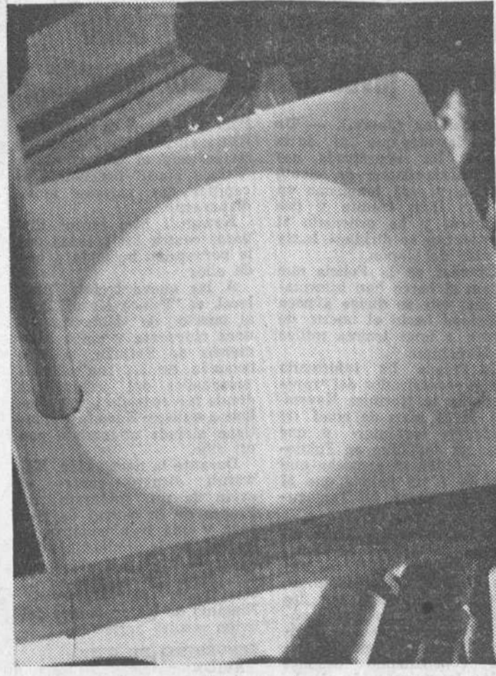
Esta es una de las fotografías que se tomaron durante el paso del planeta Mercurio por delante del disco solar. En ella se pueden apreciar algunas de las minúsculas manchas que aparecen en la superficie del Sol.
