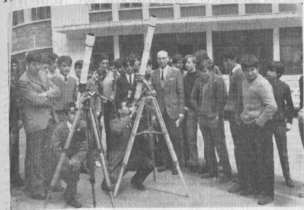
Los alumnos del Instituto Masculino de Enseñanza Media de nuestra ciudad, «Conde Diego Porcelos», observaron el último sábado, dentro de las posibilidades que ofrecía un cielo cubierto de nubes, el paso del planeta Mercurio por delante del disco solar. En lo que queda de siglo, el fenómeno sólo podrá ser observado nuevamente en los años 1973 (9 de Noviembre), 1986 (12 de Noviembre) y 1993 (14 de Noviembre). En las «fotos» aparecen los alumnos con el director del Centro, don Leandro Ruiz G. de Linares y el profesor agregado de Física y Química, don Mariano Gaspar, observando el fenómeno. A la derecha, una de las «fotos» que pudieron captar del círculo solar, con las minúsculas manchas (puntos apenas perceptibles) durante el paso del planeta.
