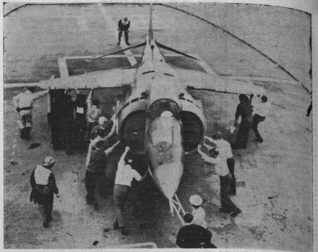
Londres. — El conjunto «Hawker Siddeley Harrier» toma tierra en el barco inglés Blake, durante las pruebas efectuadas el pasado fin de semana. Estas pruebas se efectuaron para desarrollar las actividades de estos aparatos para 1970. En la foto, hecha pública por el Ministerio de Defensa, el avión está pilotado por el jefe de pilotos de prueba de la Hawker Siddeley Aviation, Mr. Hugh Merewether. Es la primera vez que el Hawker toma tierra en un barco real. (Telefoto UPI-CIFRA)
