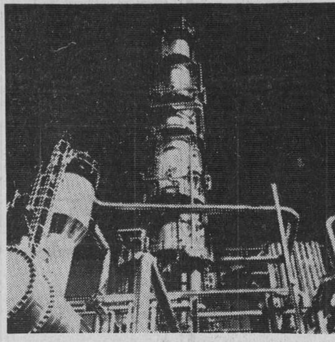
Torre de destilación atmosférica de la refinera de petróleo de Castellón. (Foto LOGOS)
