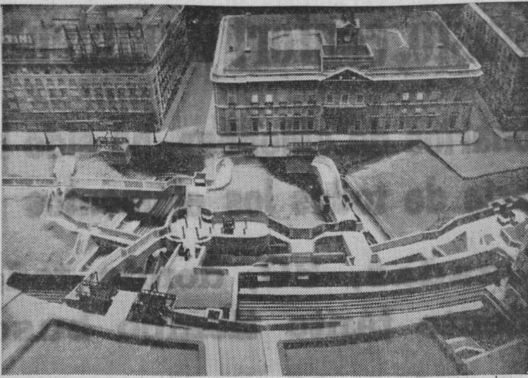
En la III Feria Internacional de la Construcción y Obras Públicas que se celebra actualmente en Madrid se muestra esta maqueta de la Puerta del Sol de la capital de España, con la distribución de las diferentes vías del Metro que discurren bajo ella. — (Foto FIEL).
