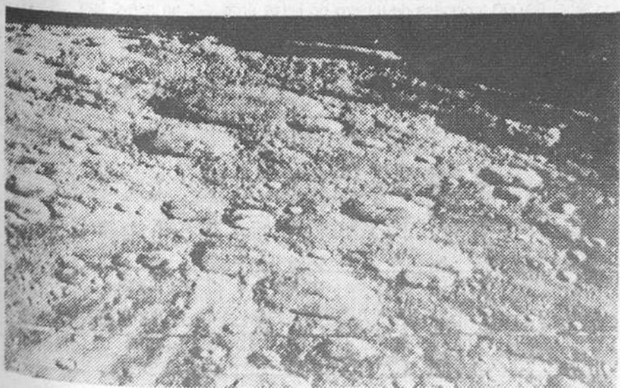
Pasadena (California, EE. UU.). — Una nueva foto del planeta Mercurio, obtenida por el «Mariner 10», en su segundo acercamiento al planeta, desde 85.120 kiló-
