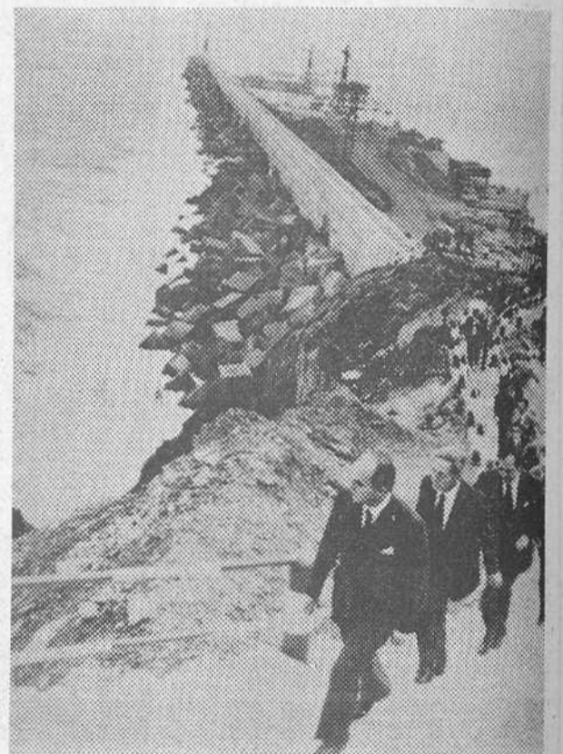
Bilbao. — El ministro de Obras Públicas, don Antonio Valdés y González Roldán ha visitado las obras del superpuerto de Bilbao. En la foto, al fondo aprecia el dique de abrigo que tendrá una longitud de 2.450 metros de los que ya están construídos. 1.640 (Foto CIFRA GRAFICA)
