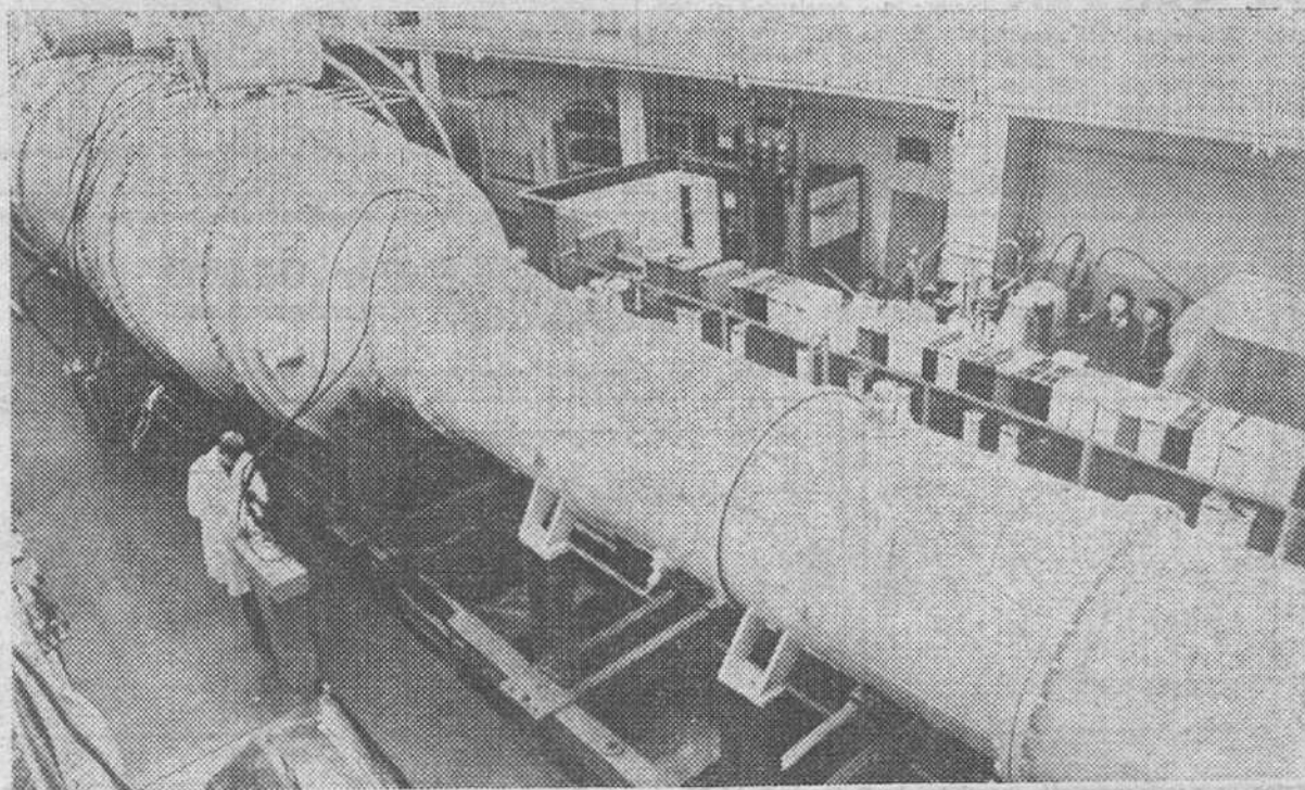
Moscú. — El primero de los 48 módulos de la instalación nuclear "Angara-5" fue comenzado a construir en el Instituto Nuclear de Kurchatov. Esta instalación será la más grande en la Unión Soviética. — (Foto EFE).
