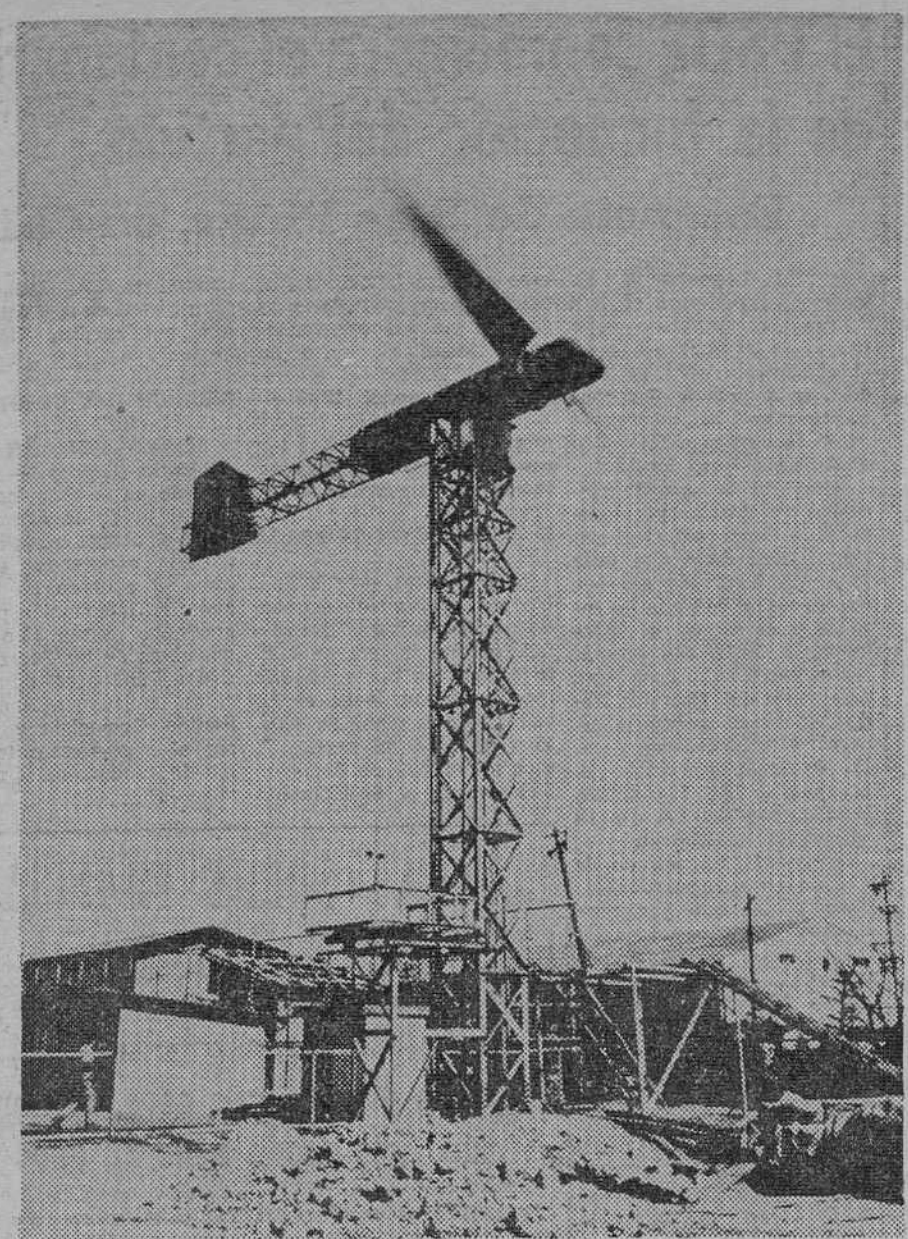
Motor eólico instalado en Japón. — (Foto FIEL-EFE)
