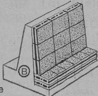
(B) aislamiento y drenaje de suelos con empleo de bloque poroso y recogida con el propio bloque poroso
