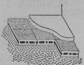
(B) aislamiento y drenaje de suelos con empleo de bloque poroso y recogida con el propio bloque poroso
