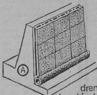
(A) drenaje trasdós de muros con empleo de bloque poroso y recogida con tubería porosa
