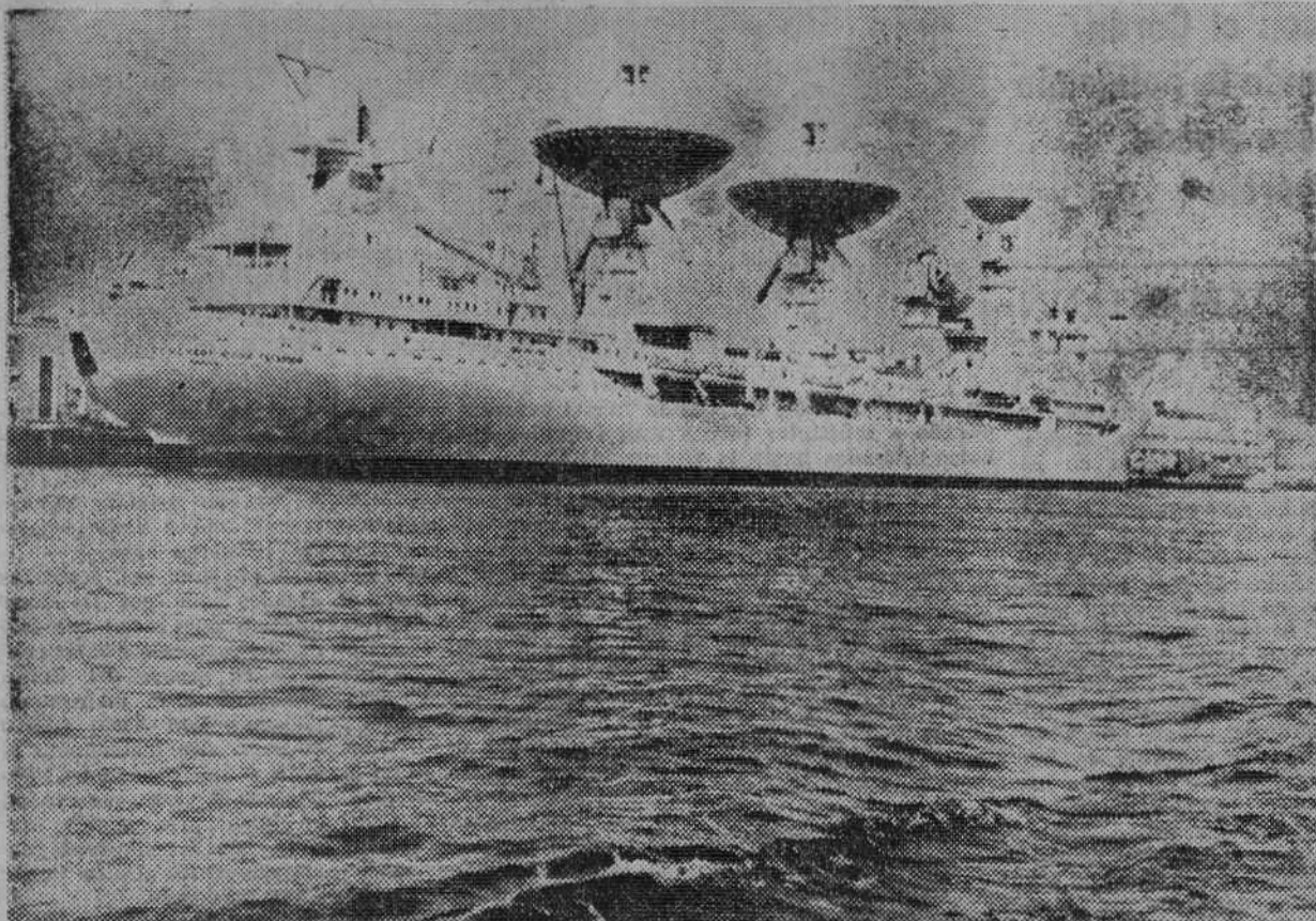
En Leningrado se ha construido el barco científico «Cosmonauta Yuri Gagarin», que pasa a engrosar la flota expedicionaria de la Academia de Ciencias de la URSS. El barco resulta ser el mayor del Mundo con 231 metros de eslora, 31 de manga y un desplazamiento de 45 mil toneladas. Va equipado con el más moderno material para el estudio de las altas capas de la atmósfera. — (Foto EFE)
