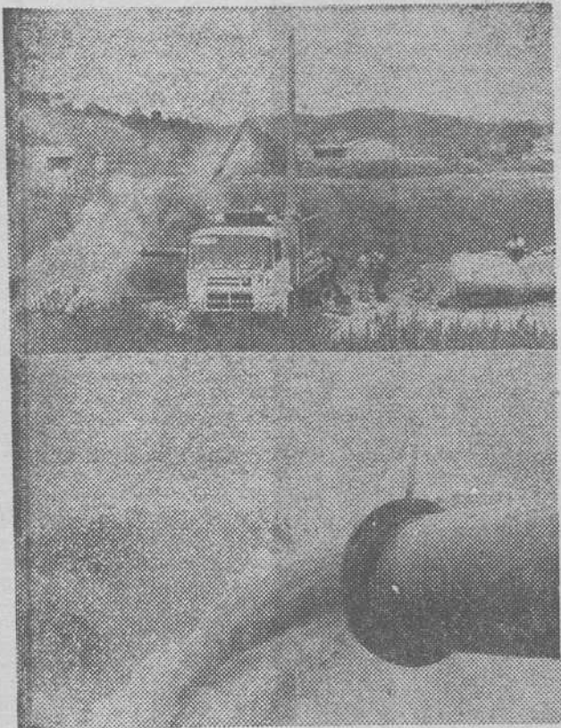
San Cugat del Vallés. — Dos aspectos de uno de los pozos del yacimiento geotérmico descubierto en el término municipal de San Cugat del Vallés, que afloran siete millones de litros de agua por día, a una temperatura de 56 grados (unas 200.000 kilocalorías). Este yacimiento puede aprovecharse para calefacción doméstica, calor industrial, invernaderos e incluso producir energía eléctrica. (Telefoto CIFRA GRAFICA)
