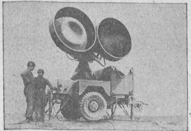
El ejército de los Estados Unidos dispone de un nuevo tipo de radar, ciego a los objetos fijos, pero capaz de detectar y seguir los blancos en vuelo casi rasante.
