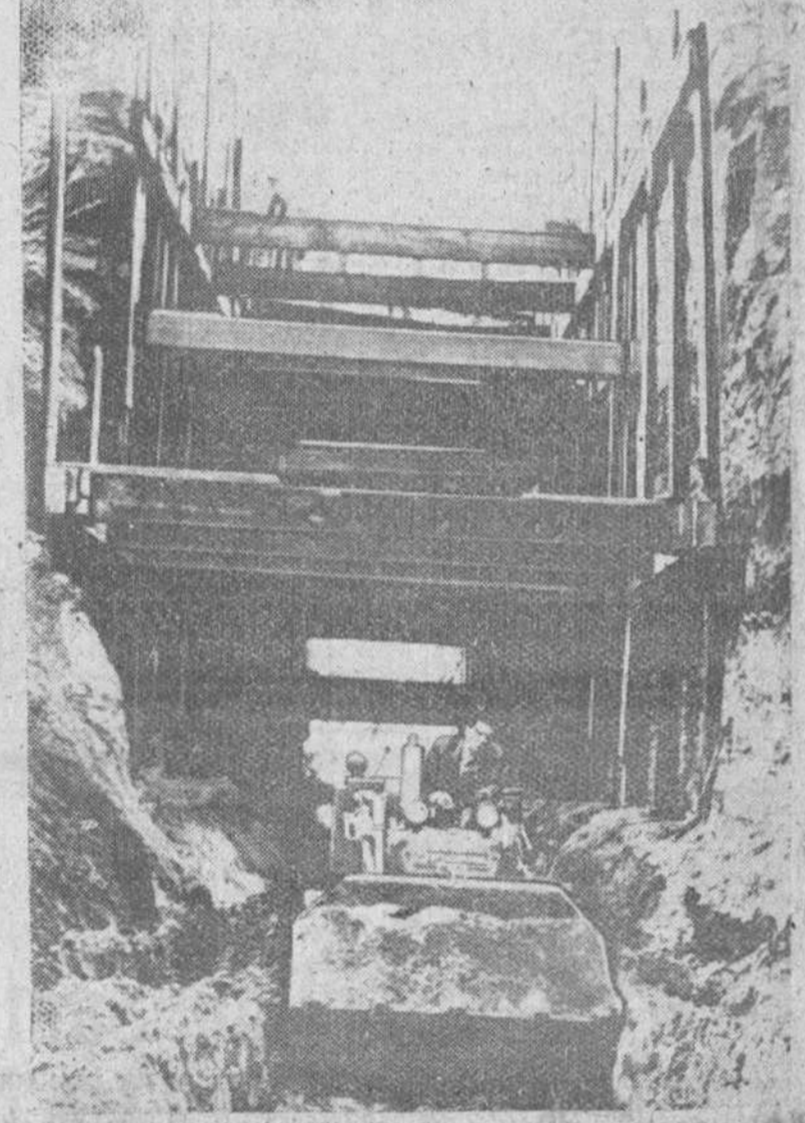
En Farnham (Inglaterra) esta máquina cortó con toda precisión un monte para permitir el paso de una nueva carretera. Comenzando desde la parte más alta, la máquina trabajó en secciones de sesenta centímetros de profundidad hasta alcanzar el nivel necesario. En pocos días de trabajo, removió y cargó en camiones, 1.500 metros cúbicos de tierra, sin equipo auxiliar alguno.—(Foto Gil del Espinar)
