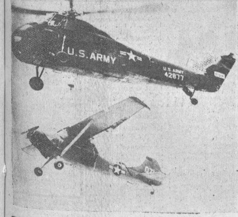
Gary (Texas). — He aquí en pleno vuelo un helicóptero 34 de las fuerzas aéreas norteamericanas que suspende un ligero avión, tipo L-19, durante una demostración celebrada en esta base aérea. Con ello se demuestra la utilidad para diversos fines de esta clase de aparatos, cuya invención se debe al español La Cierva.—(F. Cifra)
