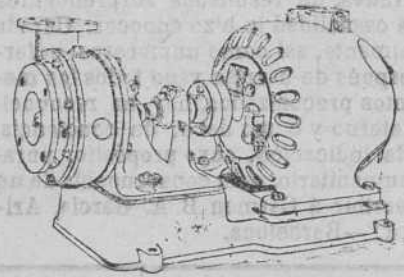
Bomba Eléctrica «Tan Gyro»
