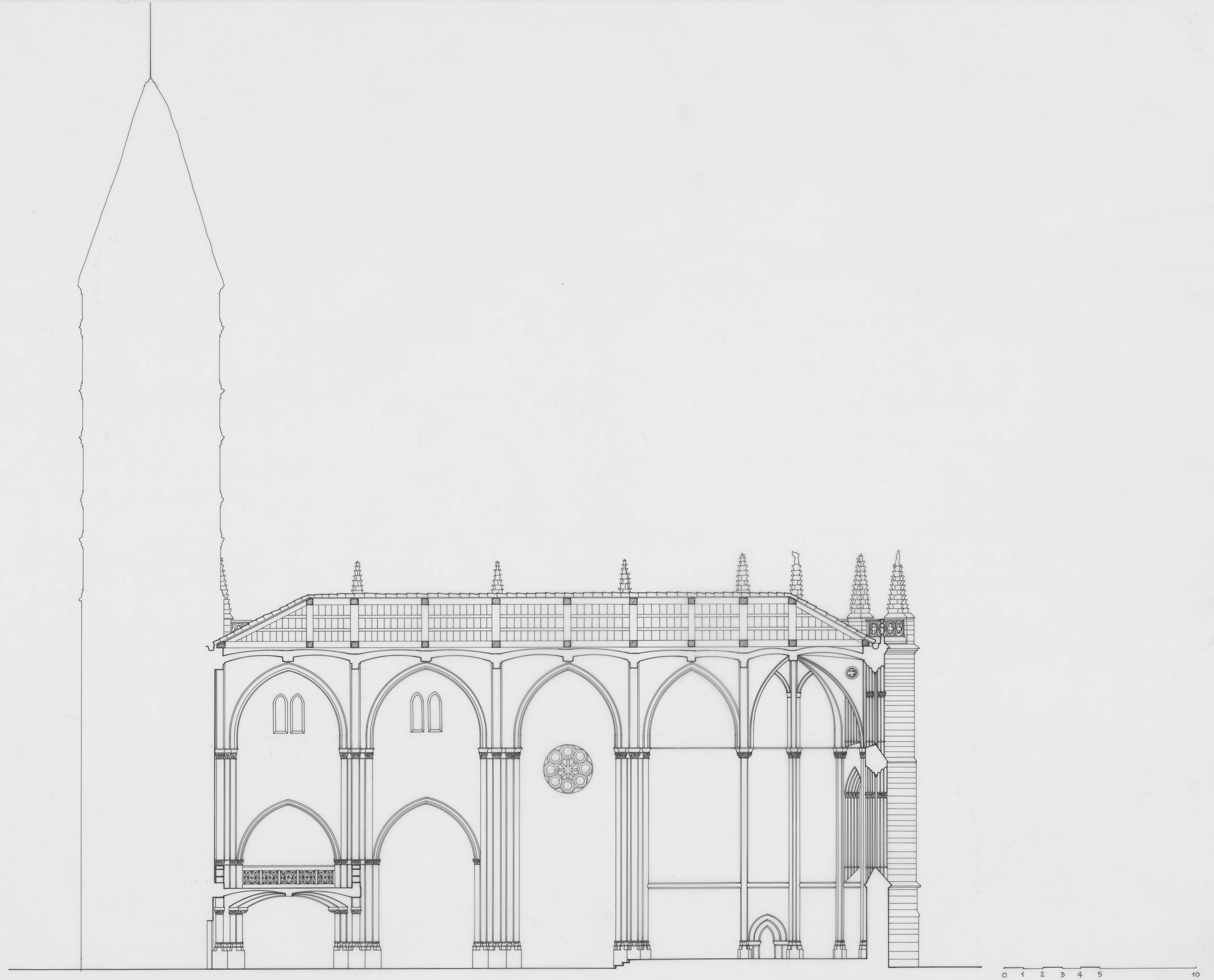
STA MARÍA DE LA ANTIGUA. VILADOLID. ESTADO ACTUAL. SECCION LONGITUDINAL. ESCALA 1:100. JULIO /91.
