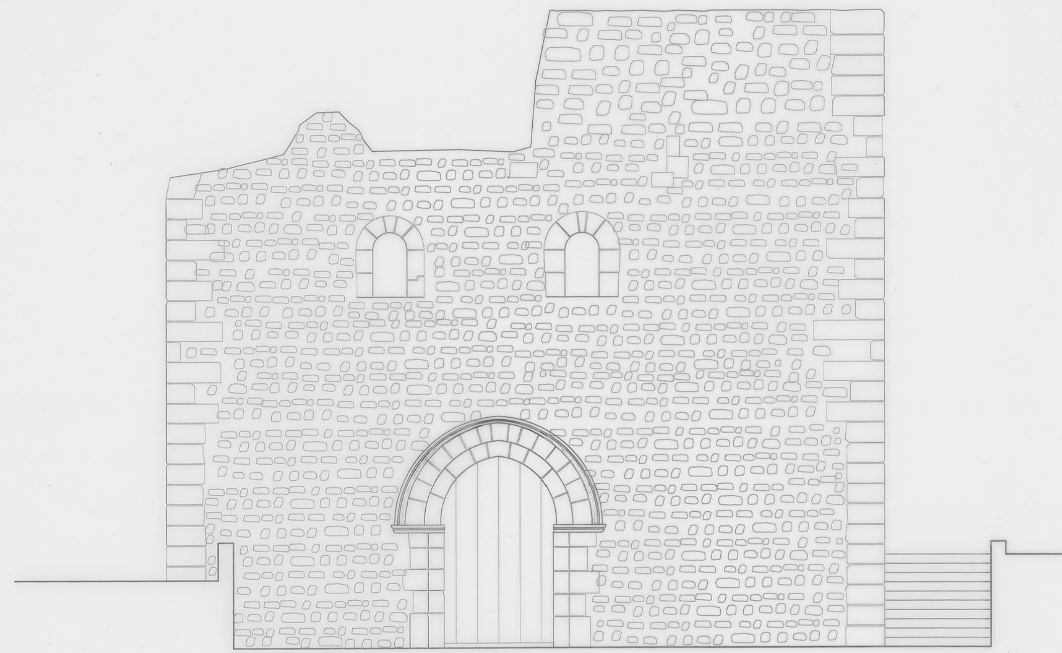
ALZADO OESTE
