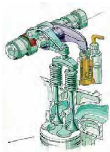
Esquema del freno motor
