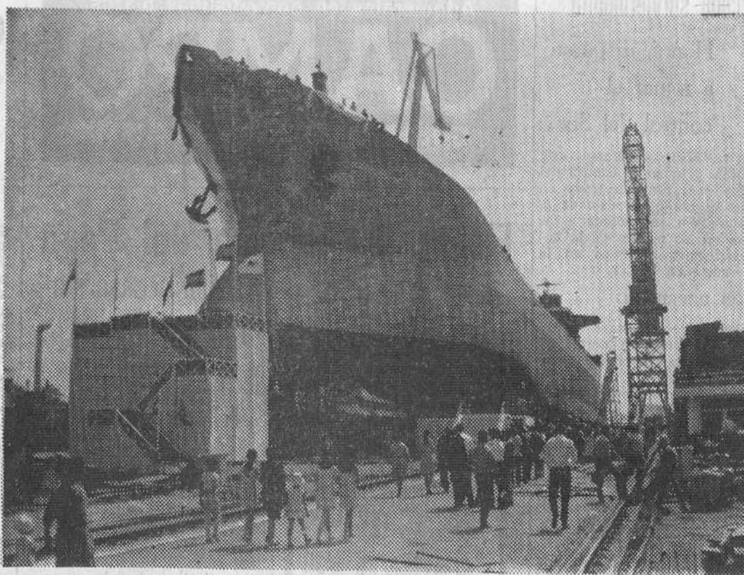
En las factorías de Matagorda, en Cádiz, ha sido botado el buque petrolero "Campomayor", de 44.000 toneladas, para la Compañía Arrendataria del Monopolio de Petróleos. Tiene una eslora de 207,70 metros, una manga de 26,50, y un calado de 10,70. — (Foto Fiel)
