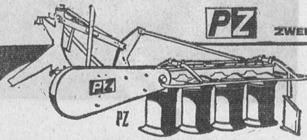
PZ ZWEEGERS & ZONEN GUADANADORA ROTATIVA PZ guadanaadoras rotativas, rastrillos, hileradores, distribuidores de abono
