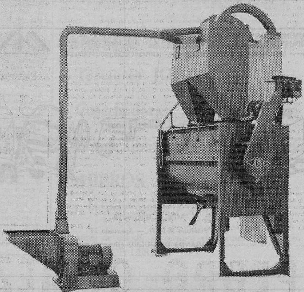
Conjunto de molino y mezcladora horizontal
