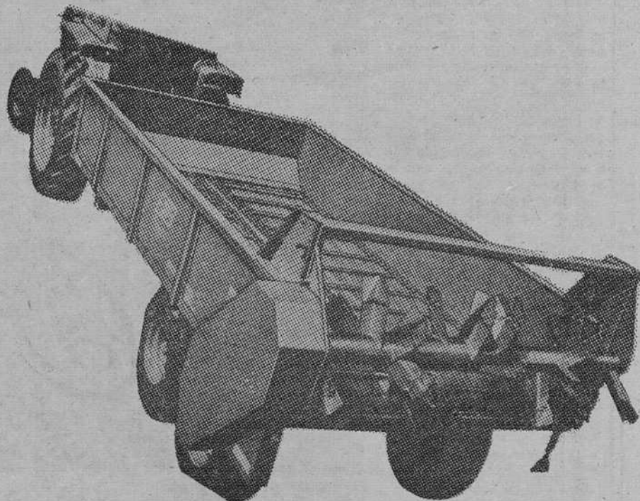
SUPERTRANSPORTE TIPO «ST 90» DE 9.000 KILOS
