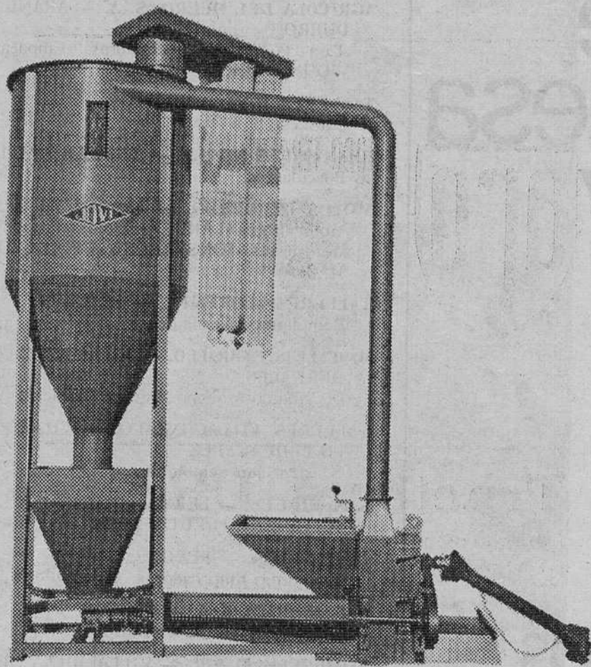
Conjunto de molino y mezcladora vertical
