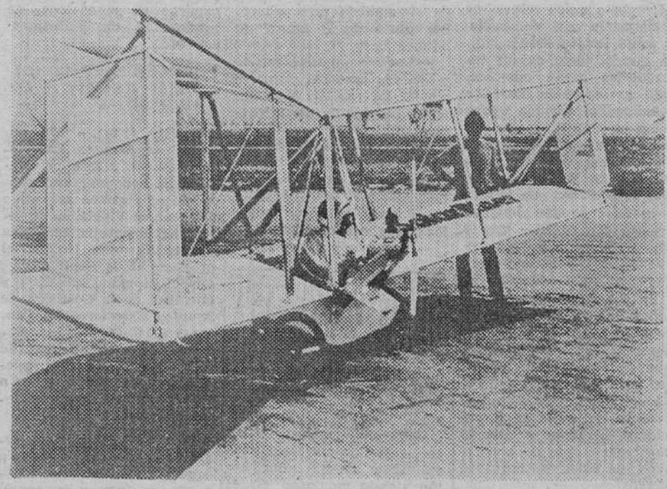
Larry Mauro, con su avioneta equipada con paneles solares, poco antes de iniciar su histórico vuelo. — (Foto FIEL-EFE).
