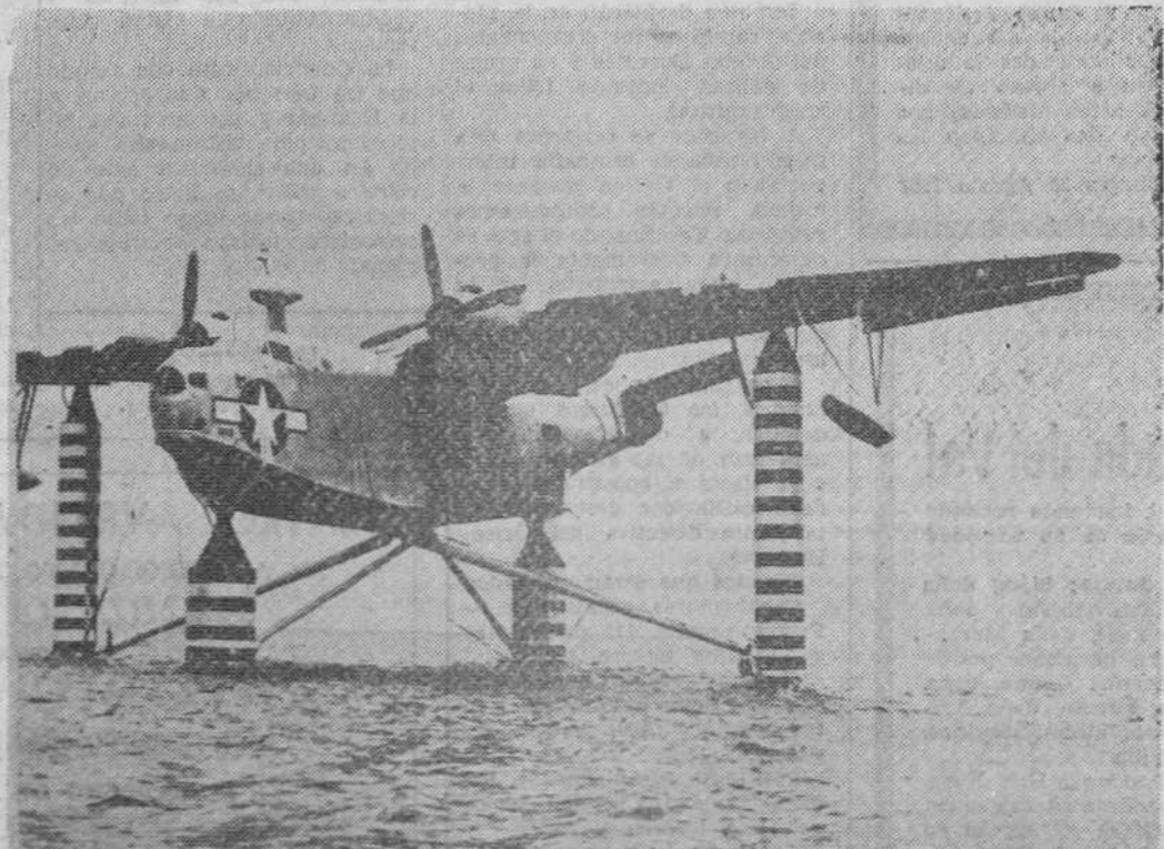
Un hidroavión antisubmarino de la Marina de los Estados Unidos, provisto de flotadores verticales, durante las pruebas realizadas en aguas de California para dotar a este tipo de aviones de un medio que les impida cabecear con el oleaje durante su acción antisubmarina. Hasta ahora las tripulaciones se veían enojadas en su cometido por el oleaje. Los flotadores se espera que puedan convertirse en retráctiles y alojarse en el fuselaje.
