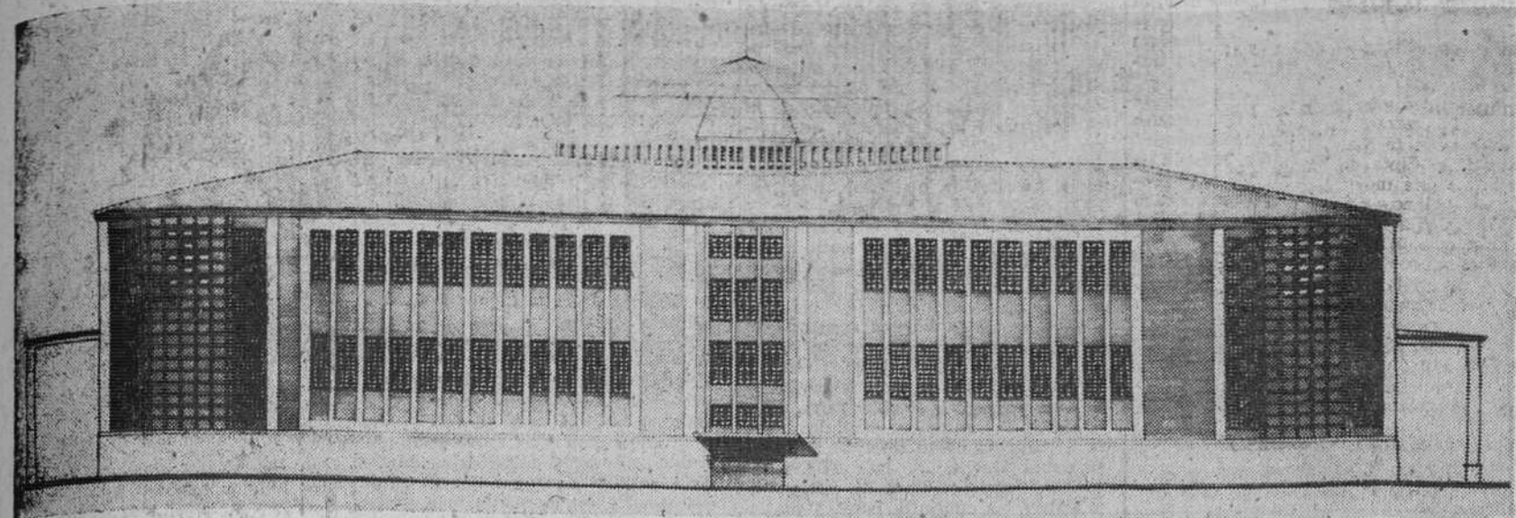
Fachada posterior del nuevo mercado de abastos. — (Reproducción fotográfica de "Fede")
