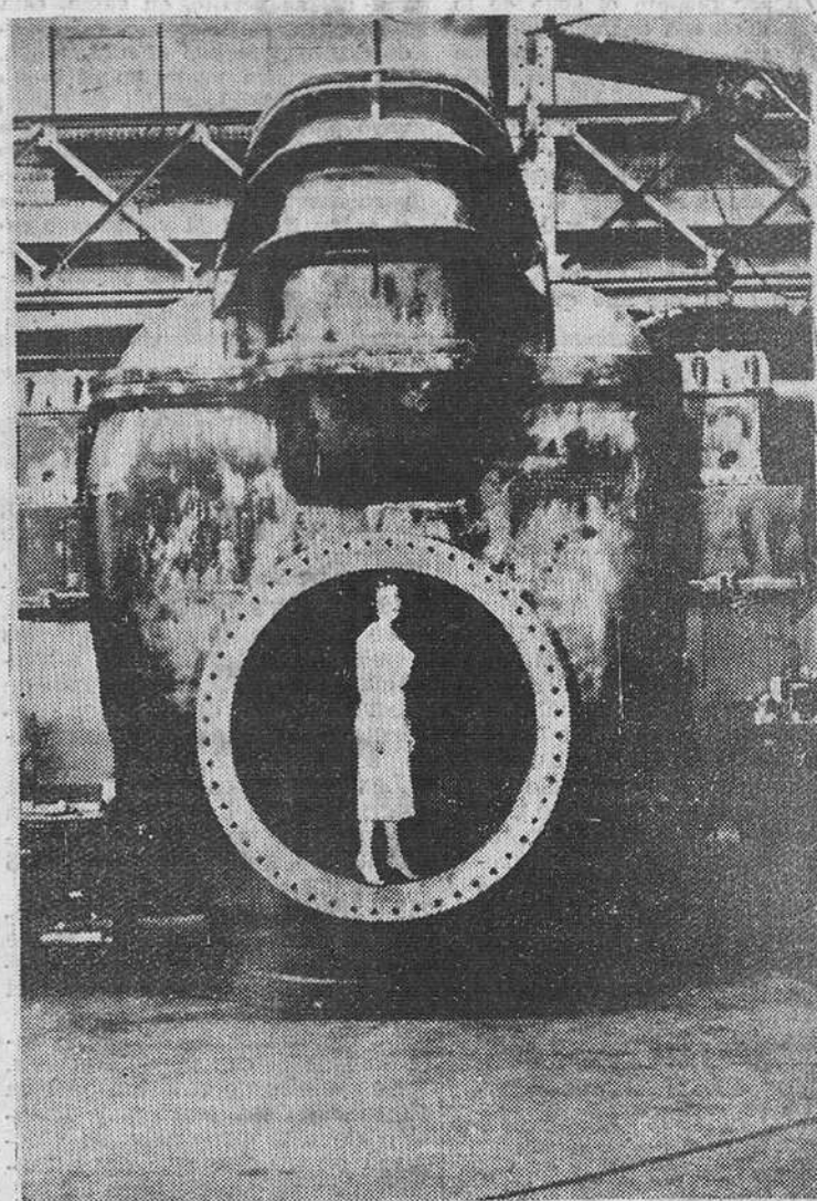
La mayor bomba de cuantas se han fabricado hasta la fecha en el mundo, con un peso de 80 toneladas, acaba de ser terminada en la factoría Werthington de Harrison (Nueva Jersey). La bomba, con destino a los servicios de alcantarillado de Río de Janeiro, tiene una capacidad de un millón de litros por minuto. De las dimensiones de su embocadura da idea la silueta de la muchacha situada de pie en la misma entrada.
