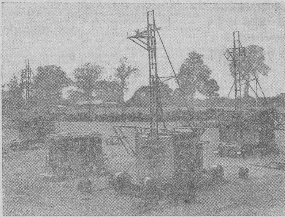
Un equipo móvil de Radar, perteneciente a un regimiento de artillería antiaérea (A. A.), compuesto por tres transmisores y un generador
