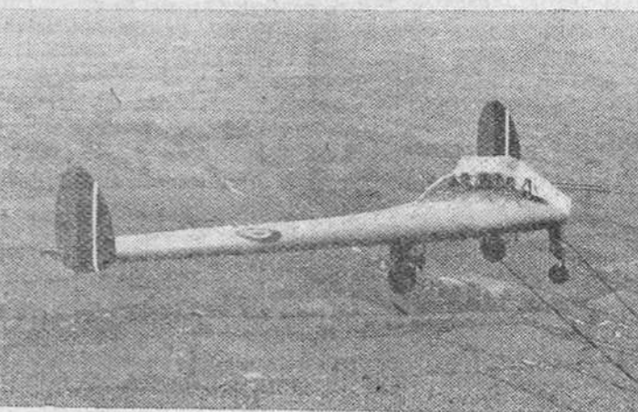
El "ala volante" es un avión creado recientemente en Inglaterra, es el aparato que posee el récord de sustentación en el espacio. Está compuesto de dos gigantes alas unidas a la cabeza de mando y carece de cola.—(Foto Calpe)
