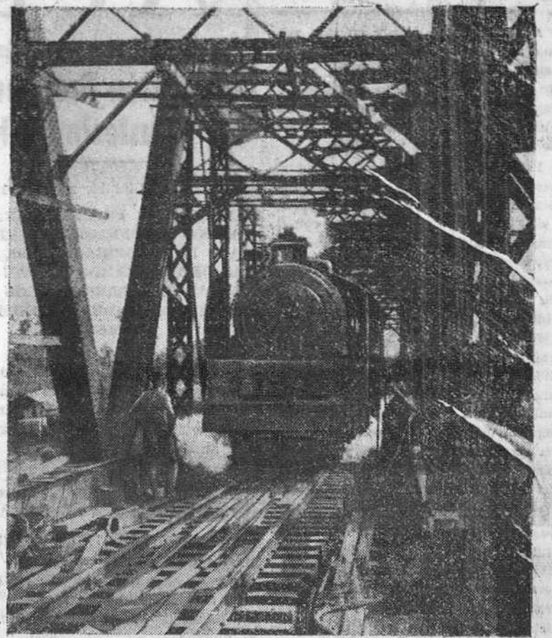
Un tren de pruebas cruza el puente de Klang, en el ferrocarril que enlaza Kuala Lumpur con Port Swettenham. Con la reconstrucción de este puente, destruido durante la guerra, que tiene 65 metros de largo, la ingeniería británica ha logrado uno de sus más grandes éxitos, pues las obras se han concluido en mucho menor tiempo que el calculado.— (Foto Calpe)
