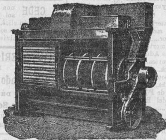
COLUMNA DESPUNTAORA
