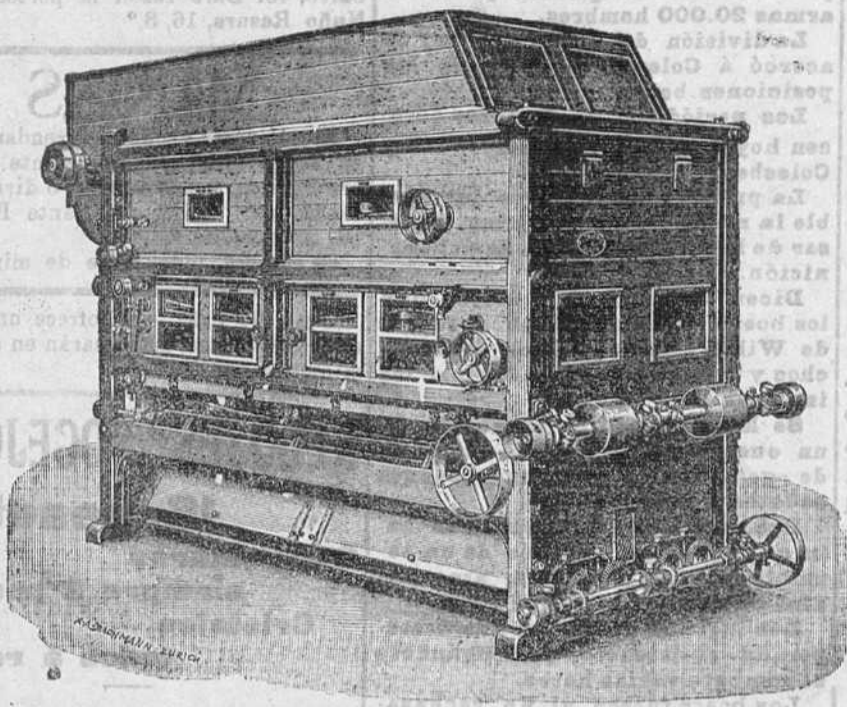
COLUMNA DESPUNTAORA
