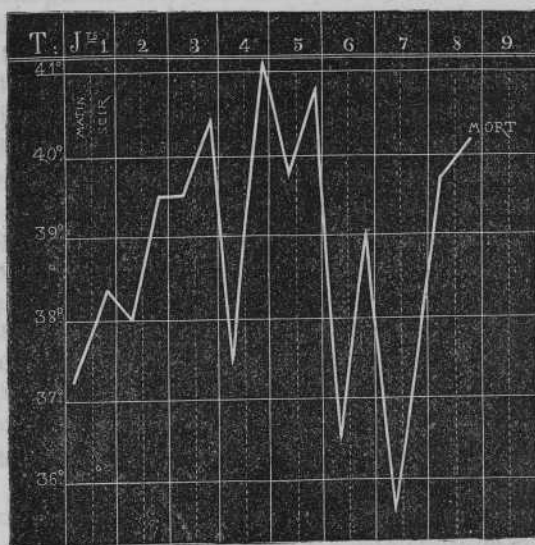
Fig 22.—Trazado de la temperatura en un caso de pihemia.
