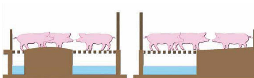
Figura 4. Suelo parcialmente enrejillado con parte sólida convexa o con pendiente, para fase de transición
