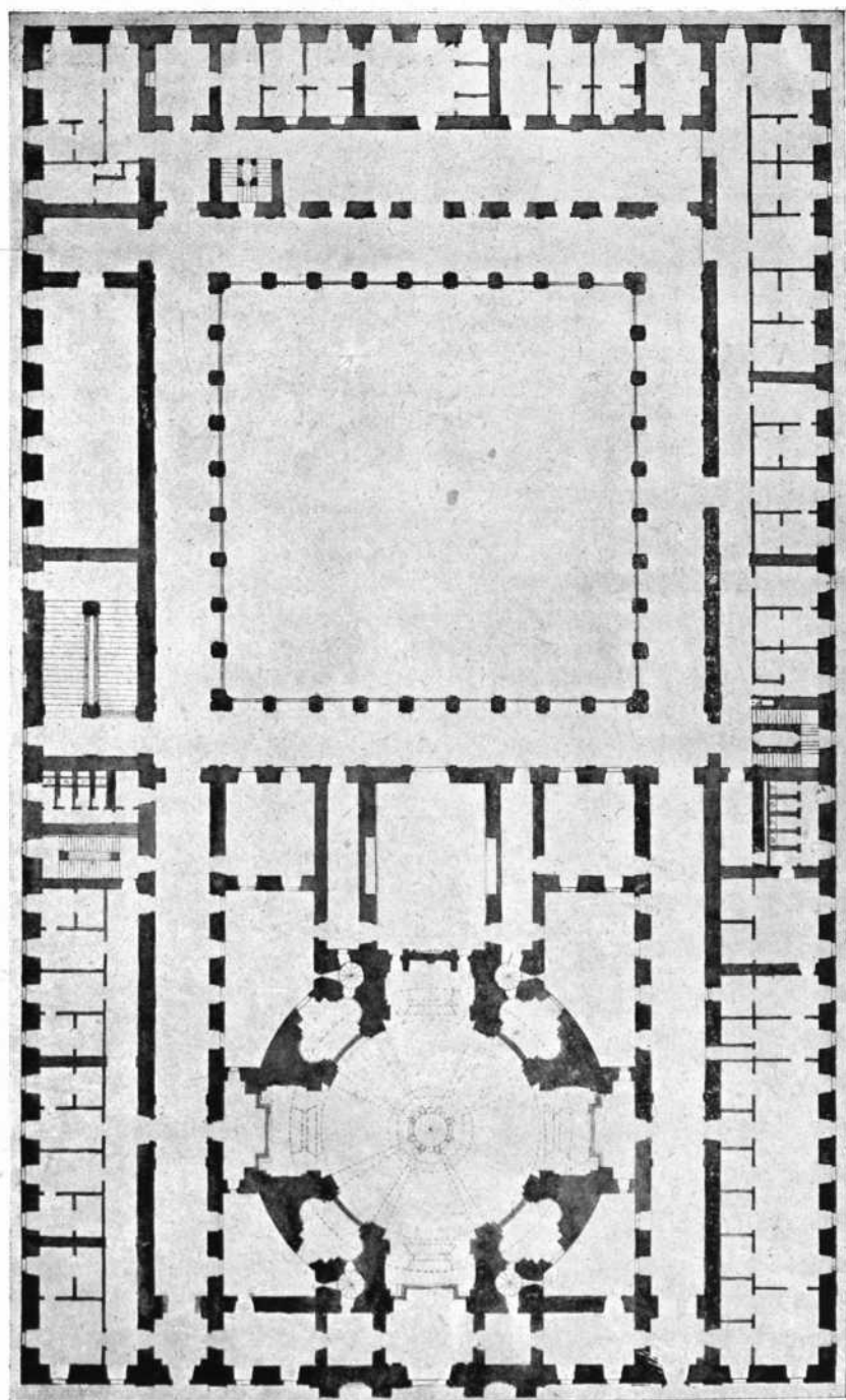
Núm. 2. Planta del cuarto bajo.
