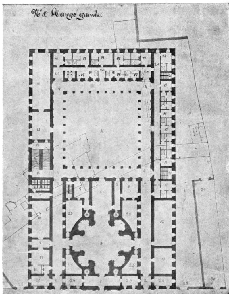
Núm. 1. Planta general y distribución del terreno.
