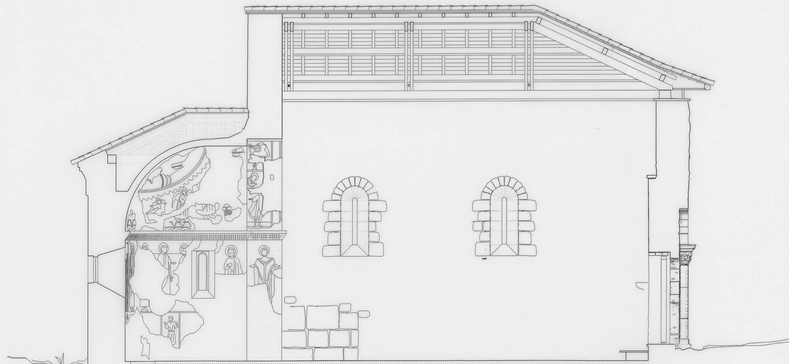
SECCION LONGITUDINAL A - A'
