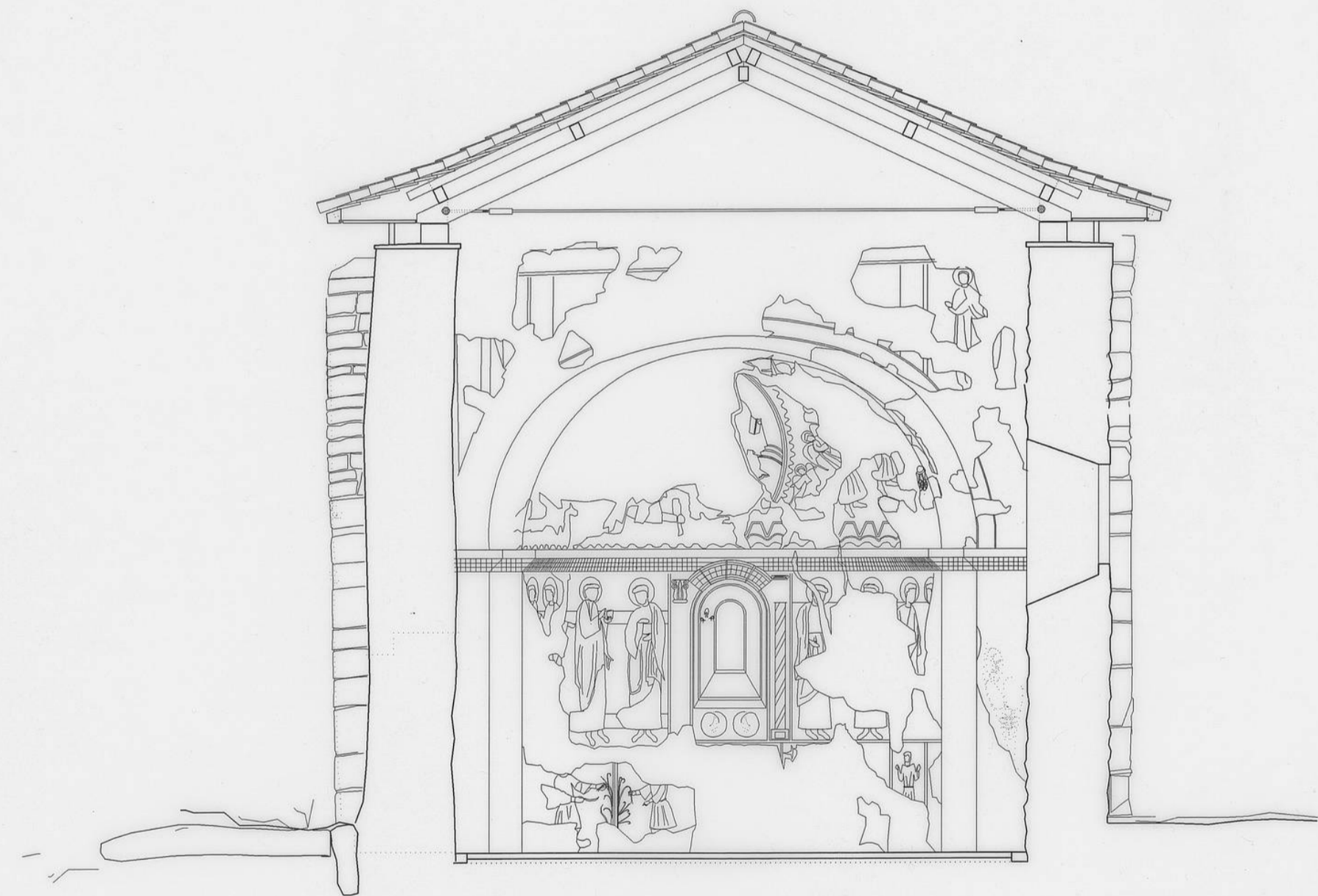
SECCION TRANSVERSAL B - B'
