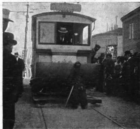
EL NUEVO APARATO SALVAVIDAS PARA LOS TRANVÍAS ELÉCTRICOS
